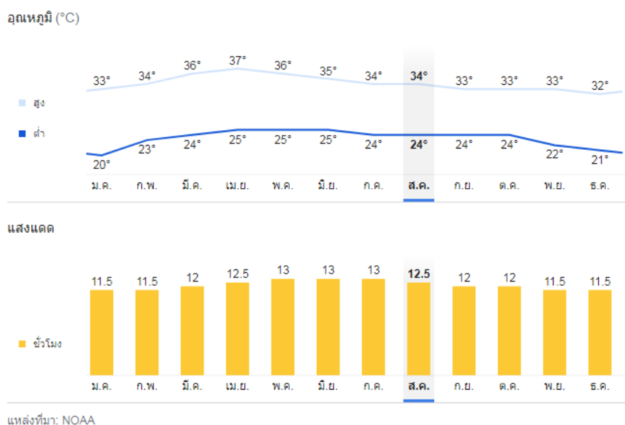
ภาพที่ ๗ แสดงค่าอุณหภูมิเฉลี่ยในรอบ ๓ ปี ตั้งแต่ ปี พ.ศ. ๒๕๖๓ - ๒๕๖๖ (ที่มา: กรมอุตุนิยมวิทยา, พ.ศ. ๒๕๖๗)
